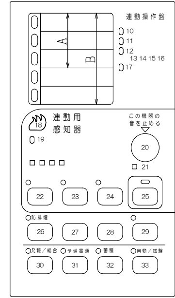
スイッチ操作部詳細図
