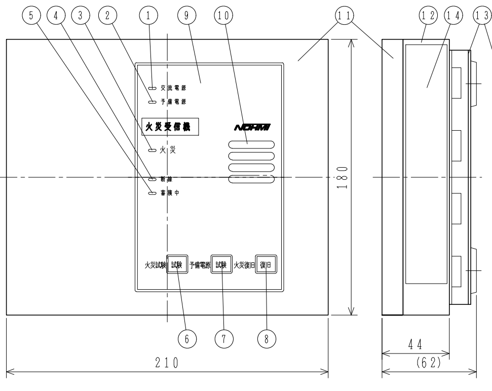
取付寸法詳細図 (正面図)
