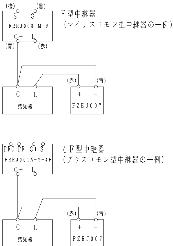
接続図
