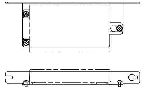
機器取付イメージ
