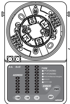
アドレス設定器 FZAJ004-P または FZA012A
