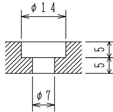
A-A断面
