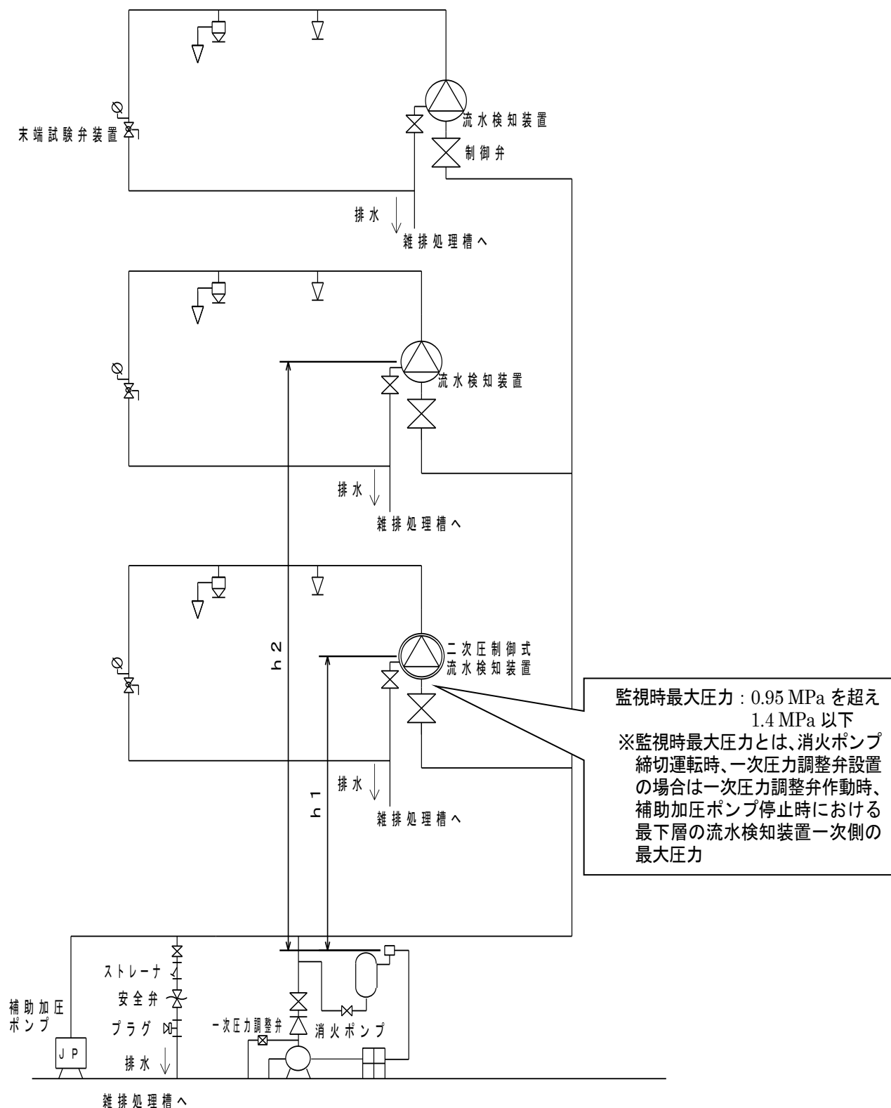
設備図 (その 2)
