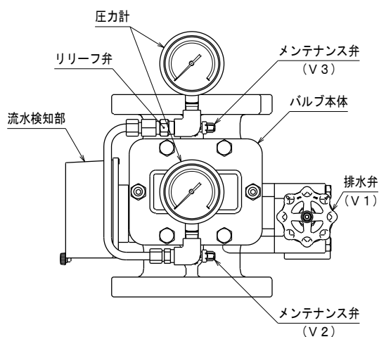
図 1. 機器外観
