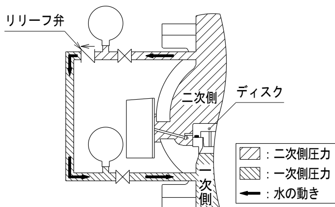
図 4. 二次側配管内圧力上昇時の水の動き
