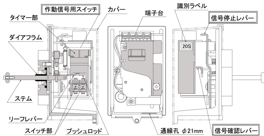
図 3. 流水検知部（端子台ボックス）詳細
