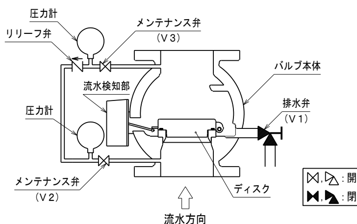
図 2. 機器系統 (監視時)
