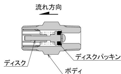
図 5. リリーフ弁詳細
