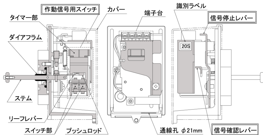
図3. 流水検知部（端子台ボックス）詳細
