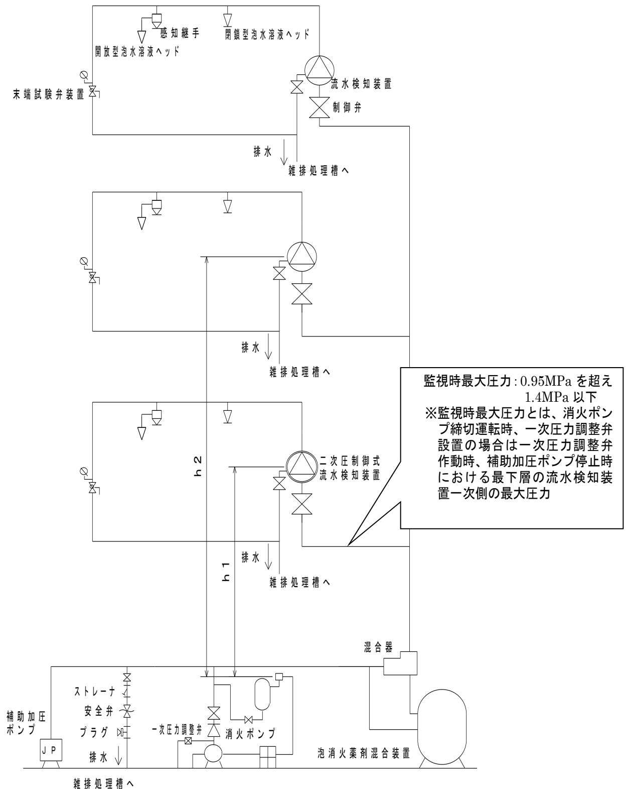
図 24 設備図 (その 2)
