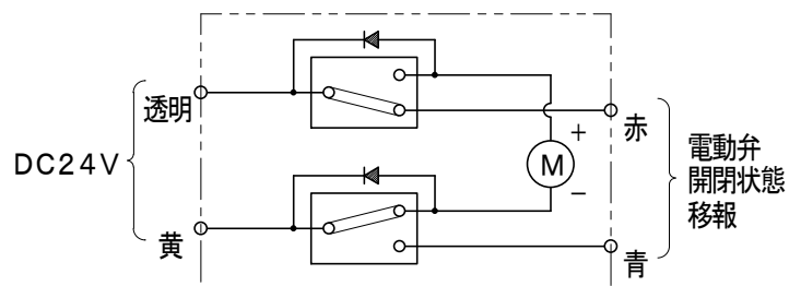
回路図 (図は閉止状態を示す)
