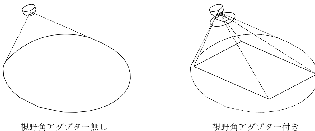
図1. 炎感知器の監視範囲
