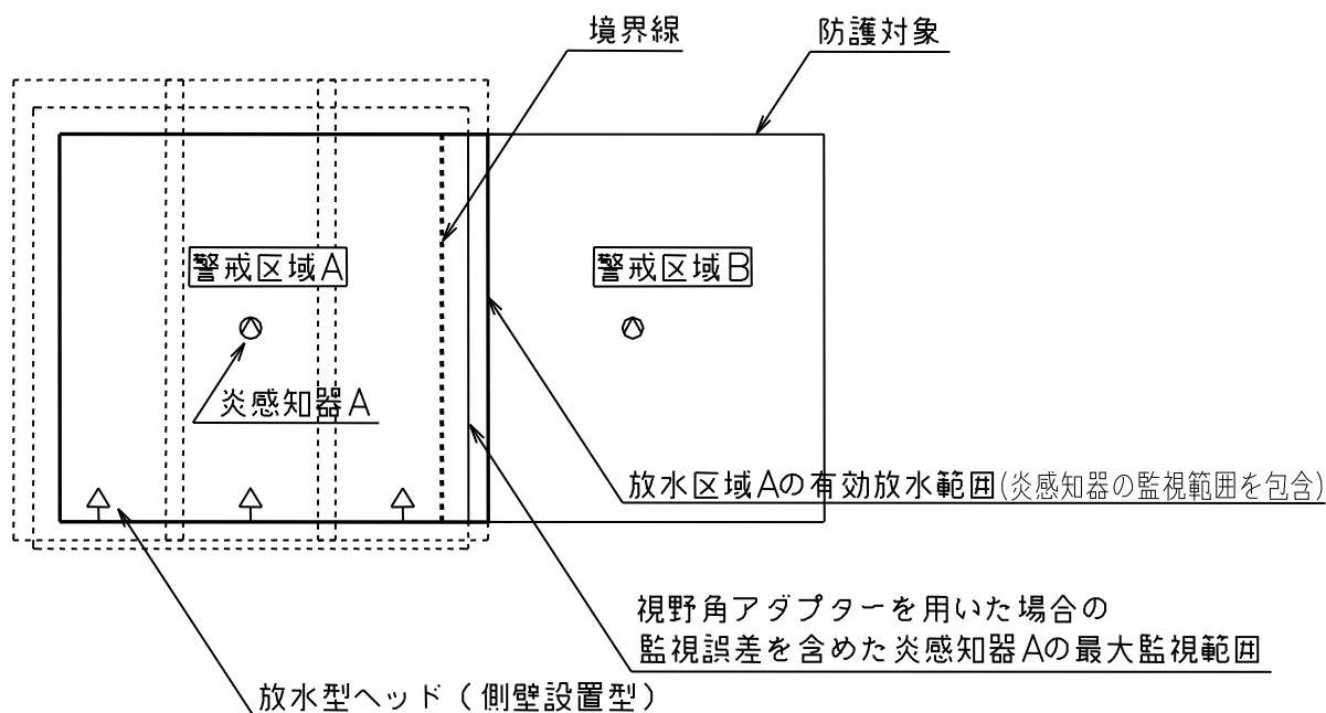
図6．視野角アダプター適用時の放水区域の設定方法
