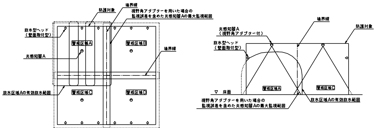
図 8．炎感知器は天井設置、放水型ヘッドは壁面設置する場合の例
