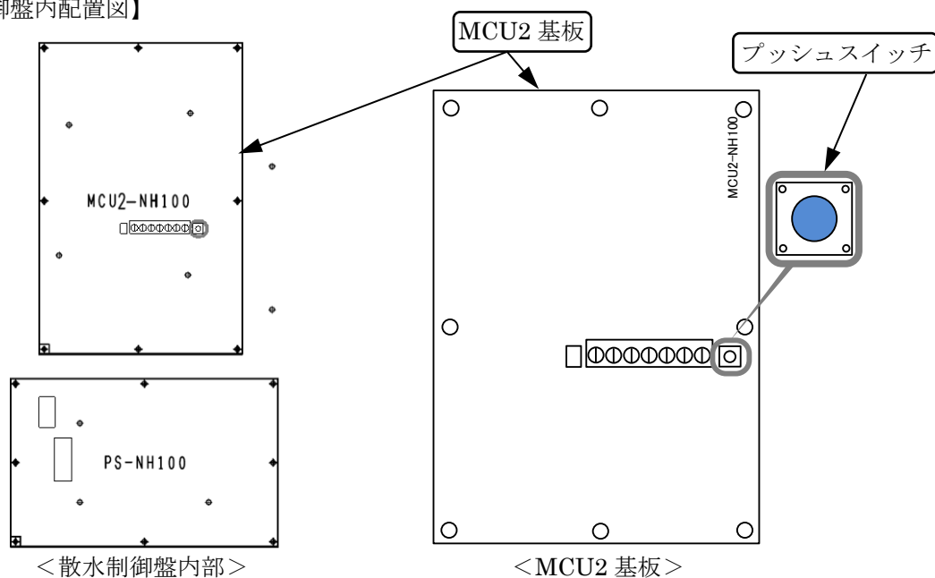
【散水制御盤内配置図】
