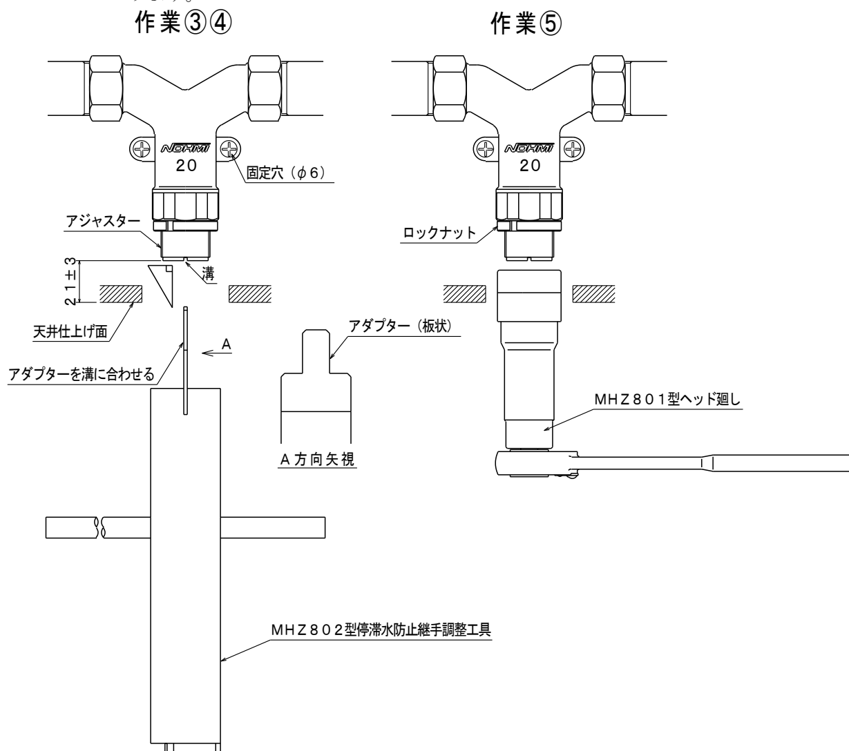
図6. 停滞水防止継手のアジャスター長さ調整（その2）
