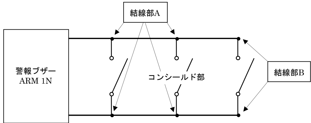
図 1 2. コンシールド部配線図
