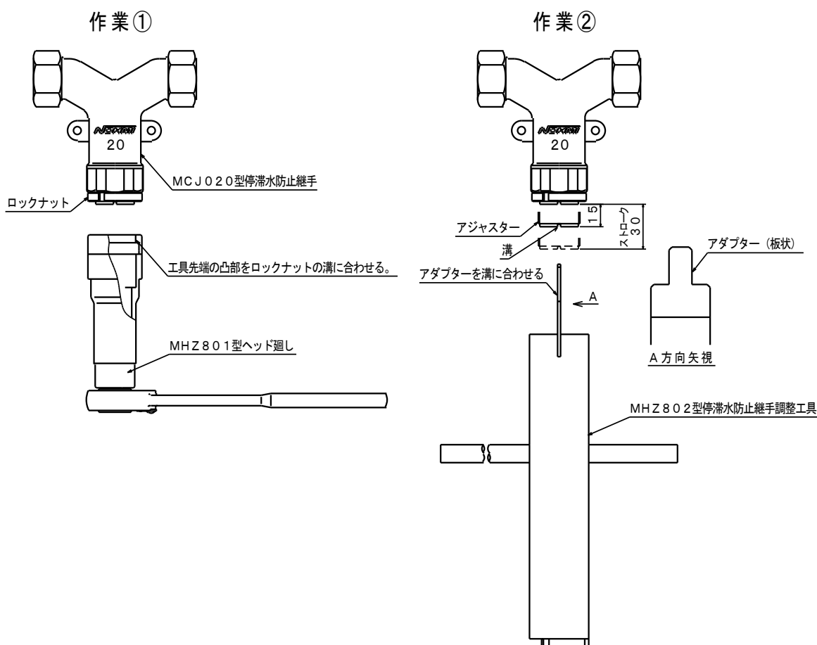
図5. 停滞水防止継手のアジャスター長さ調整（その1）
