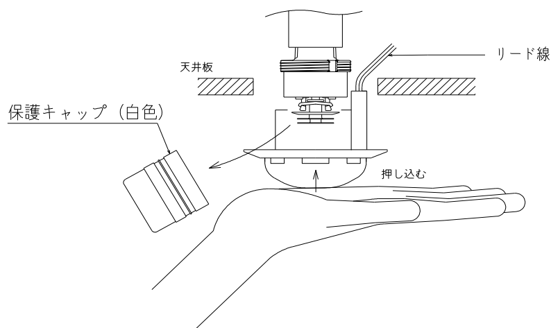
図 8. コンシールド部の取り付け
