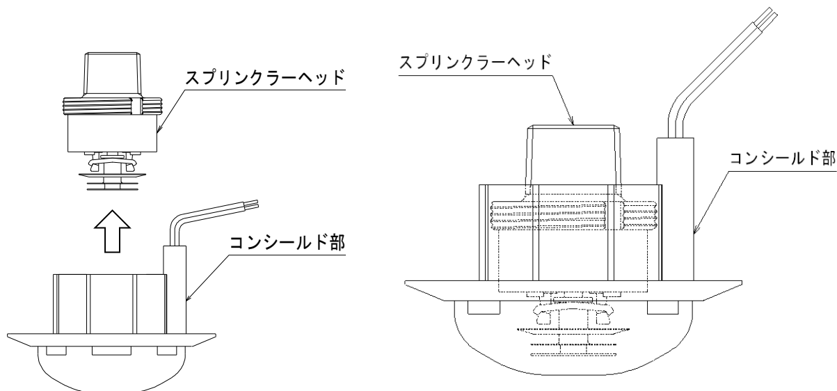
図3. コンシールドヘッド
