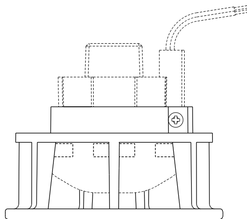
図 10. MZHJ004-P型コンシールドヘッド用保護カバー
