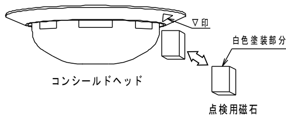
図 1 3. 点検用磁石の使い方
