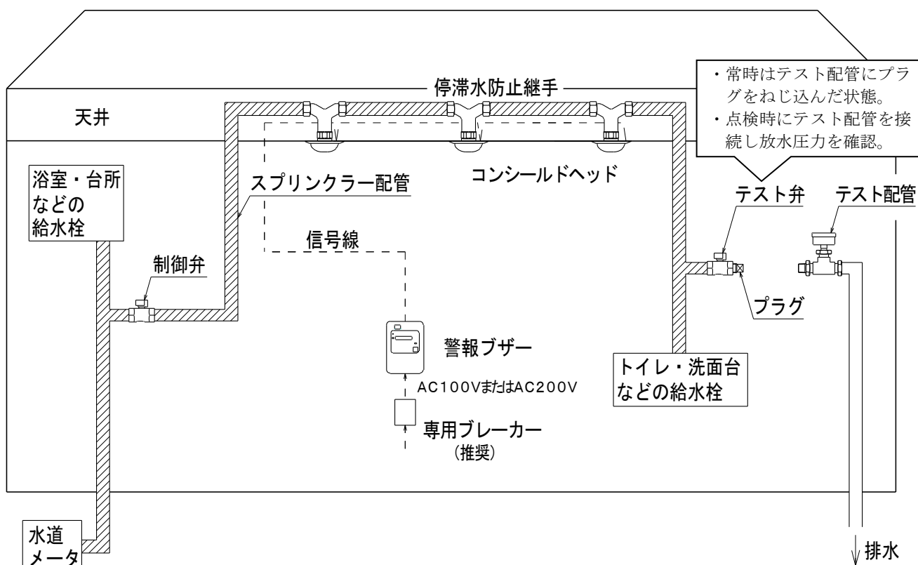
図2. システム図（例）
