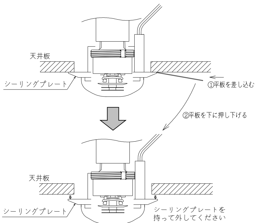
図 9. コンシールド部の取り外し
