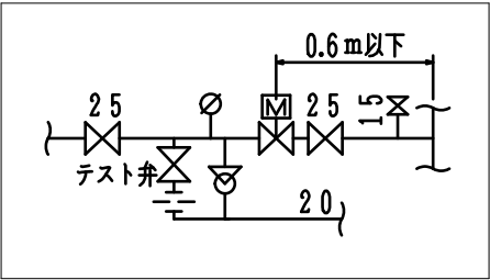
テスト弁廻り詳細図
