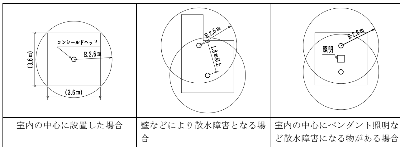
図4-1 コンシールドヘッド配置例
