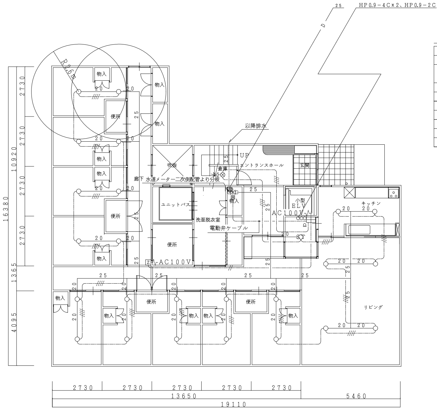
図4-9. 平面図設計例 (1階)
