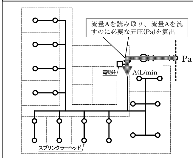
図5-3 摩擦損失計算の概要説明
