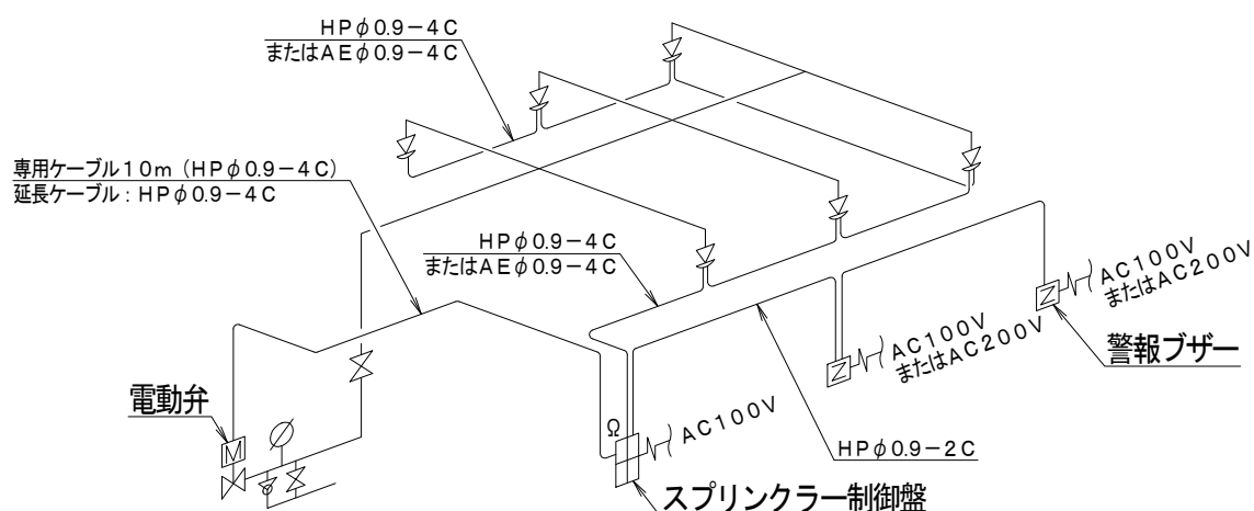
図4-7 電路配線例図
