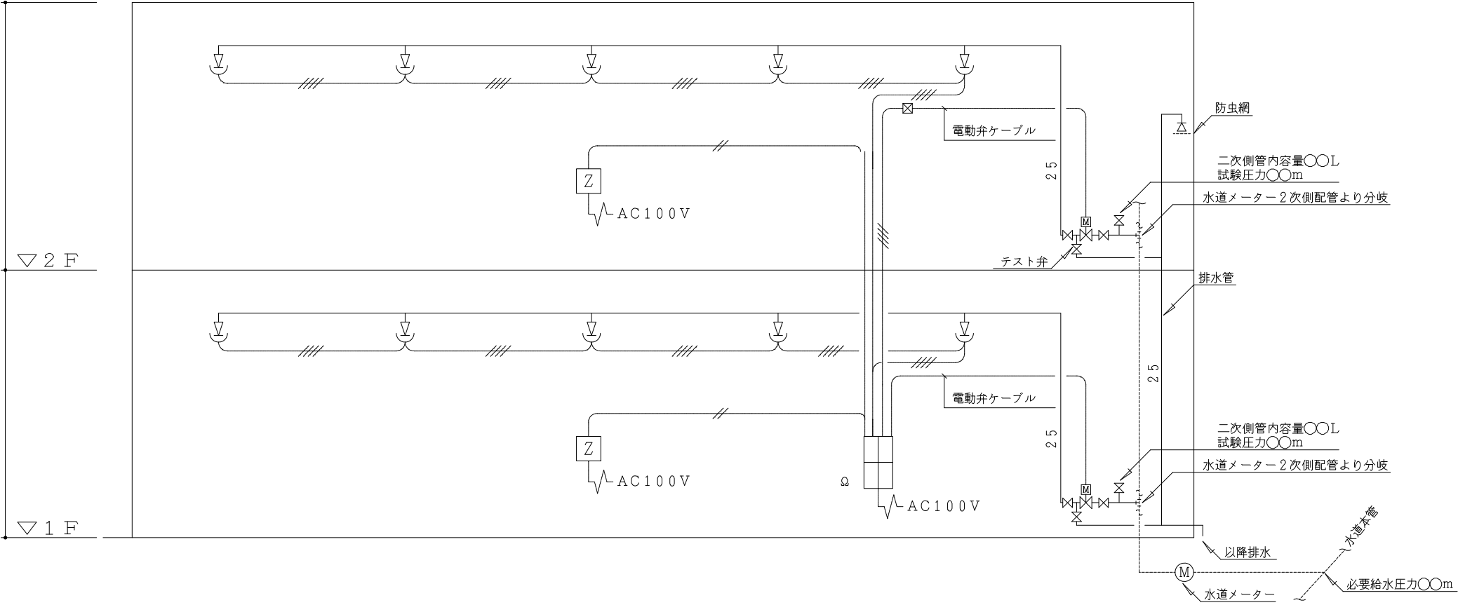
図4-11. 系統図設計例
