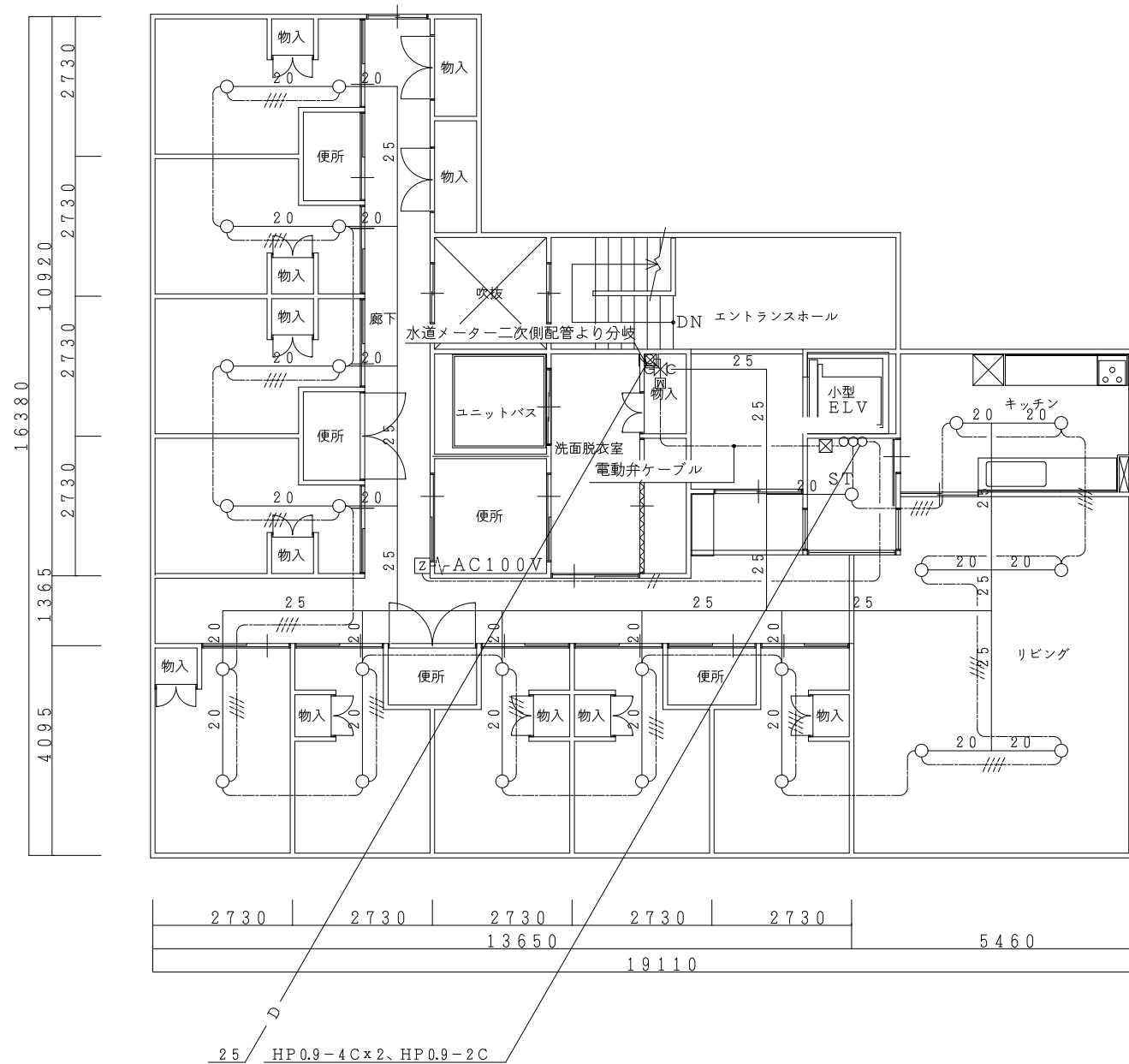
図4-10. 平面図設計例（2階）
