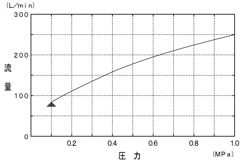
圧力-流量特性図
