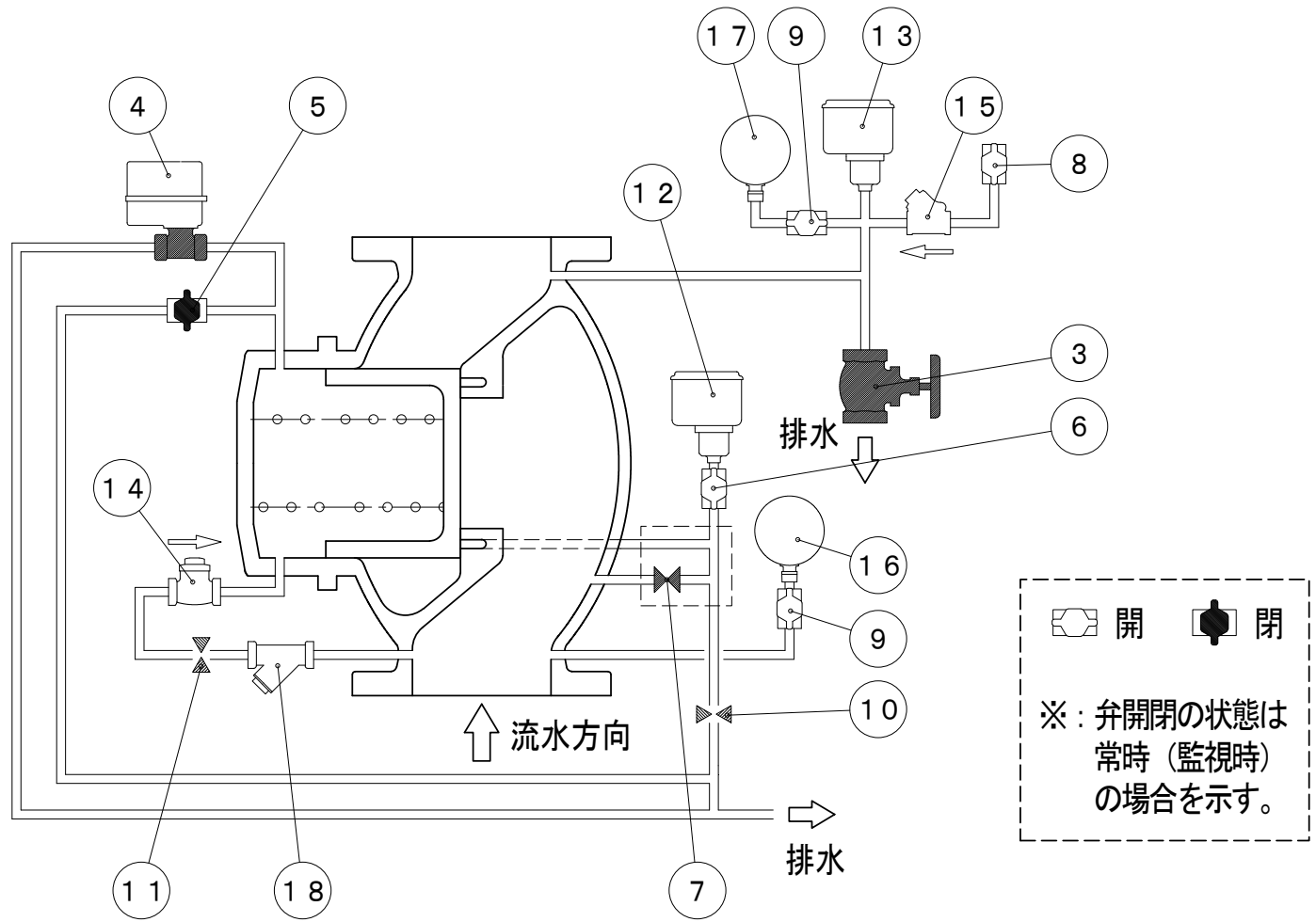
装置構成図
