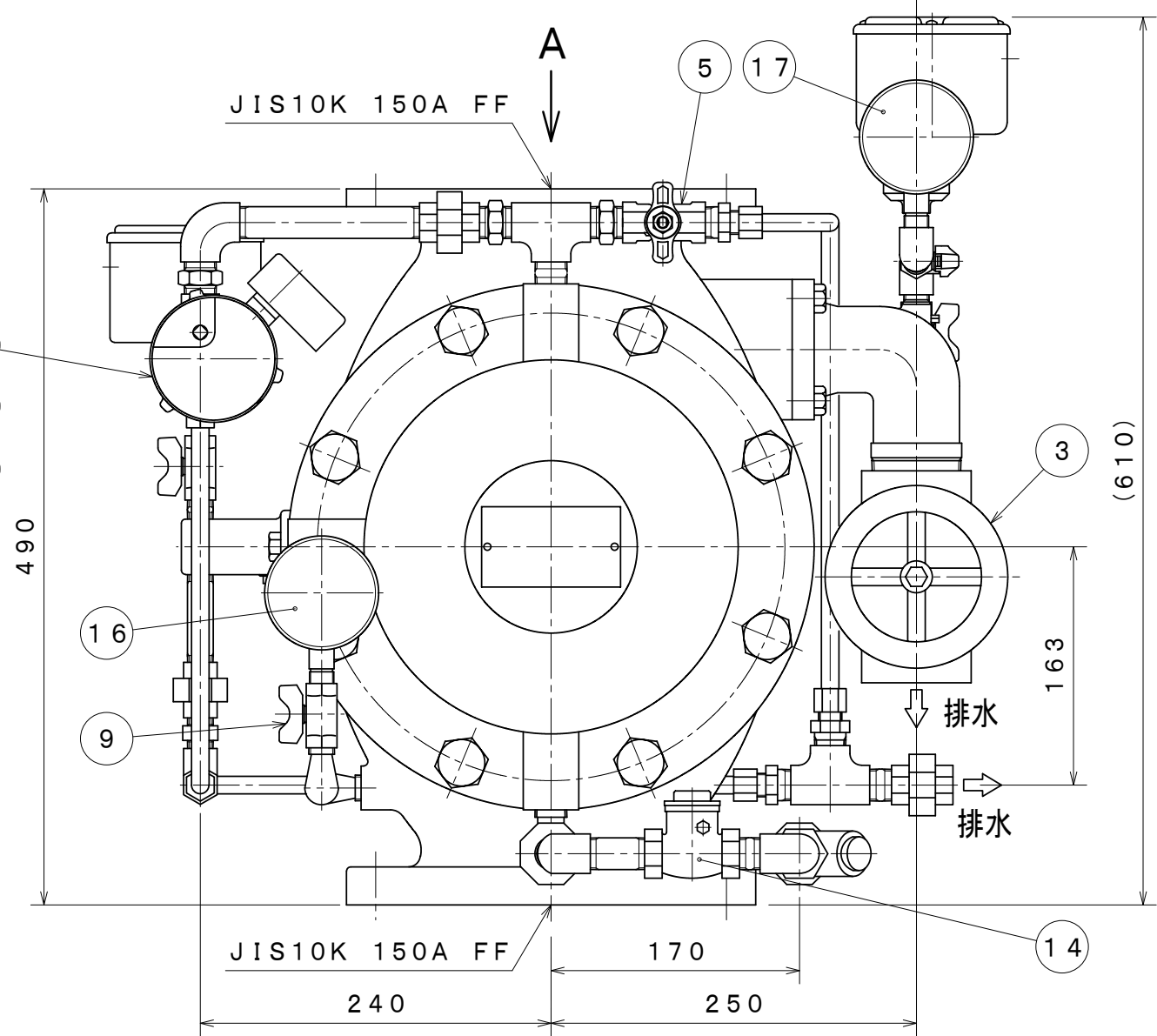
流水方向
