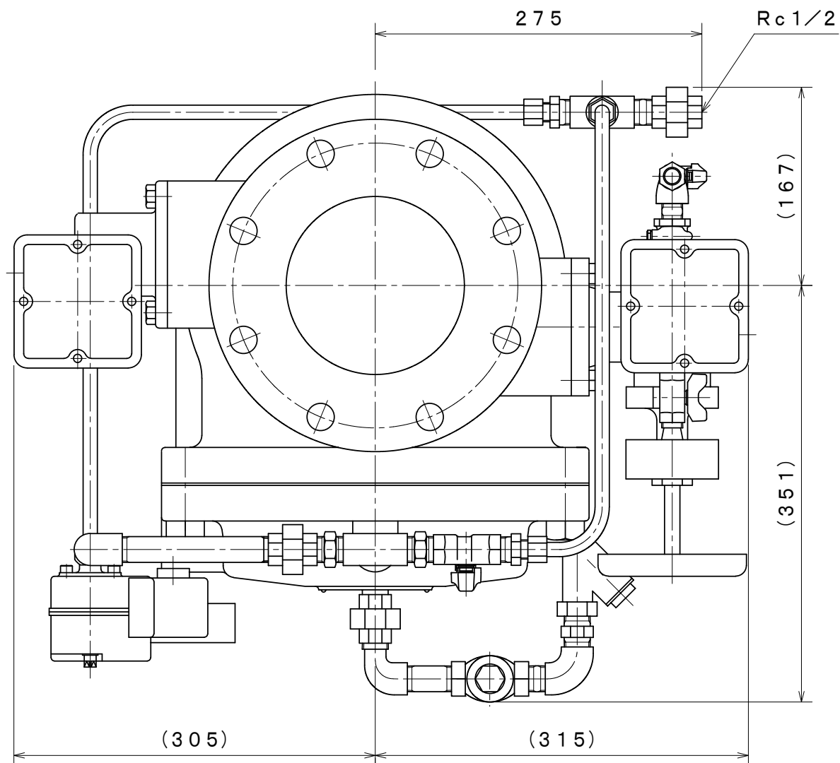
A矢视图
