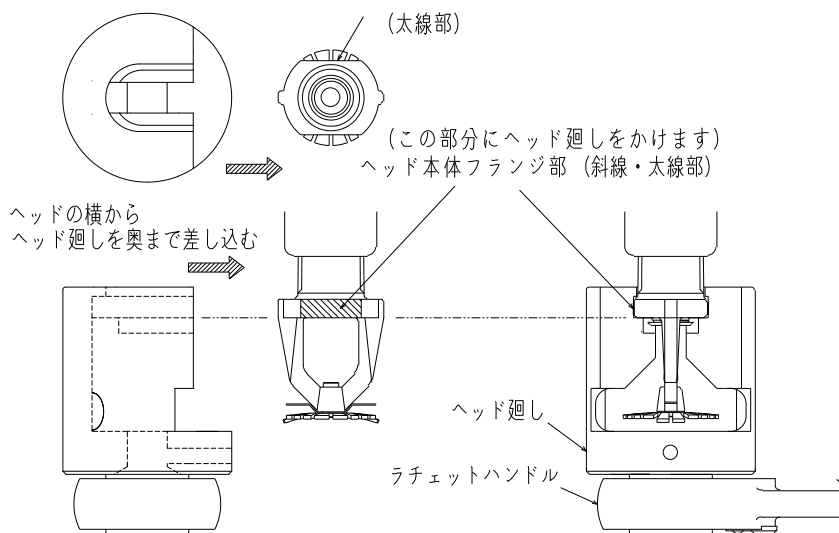
図 3. ヘッドの取付方法
