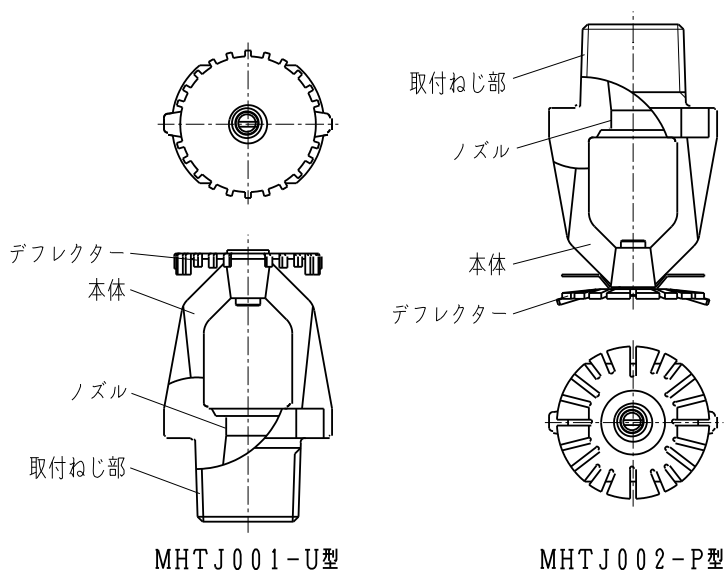
図 1. 外観図
