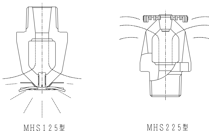
図 2. 作動状態図
