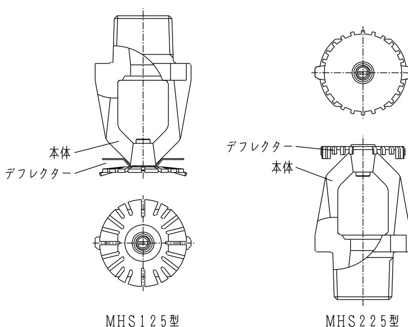
図 1. 外観図
