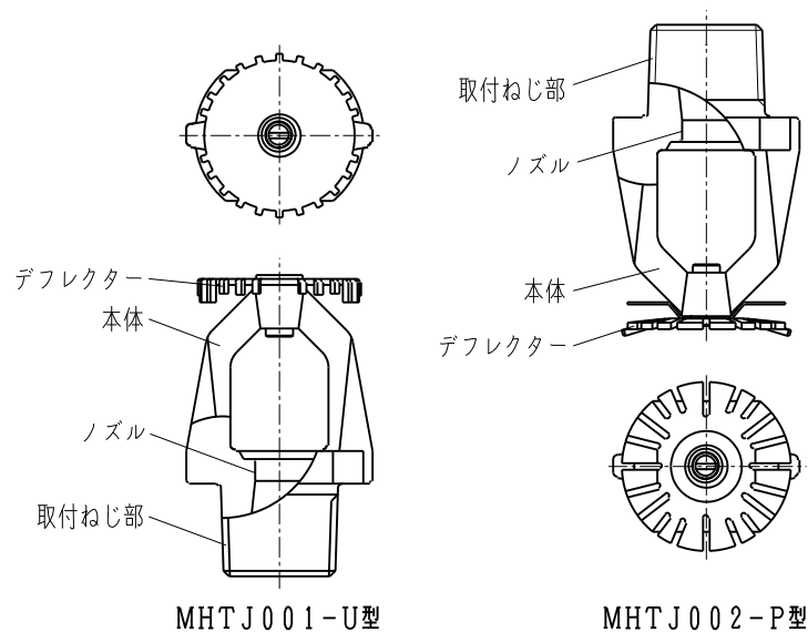
図 1. 外観図
