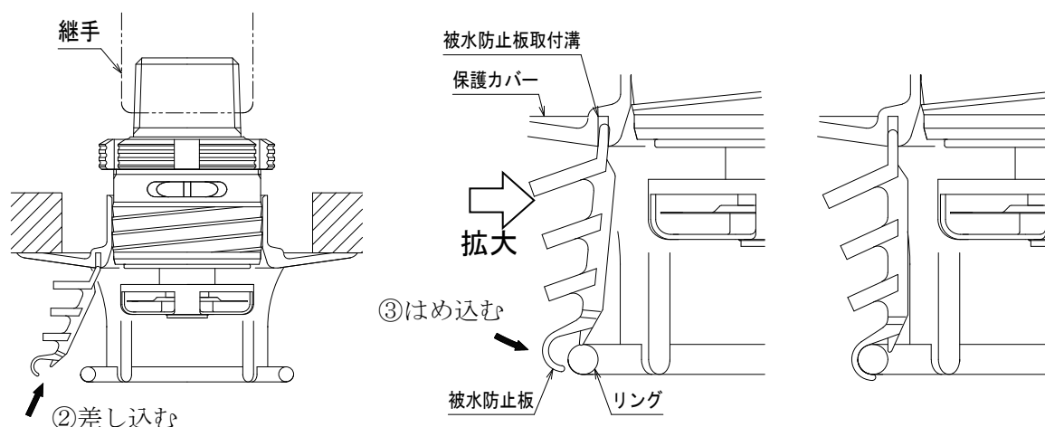
図 12. 被水防止板の取り付け（その 1）
