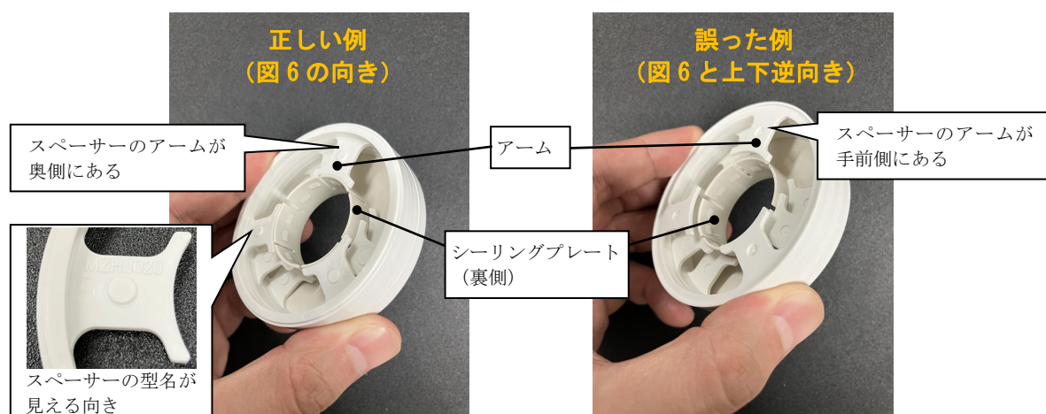
図 9. スペーサーの向きと組み付け状態
