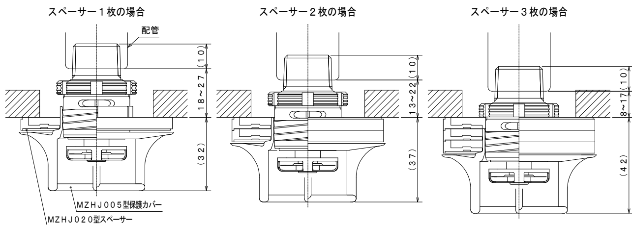
図 11. スペーサー使用時の取り付け状態（保護カバー）
