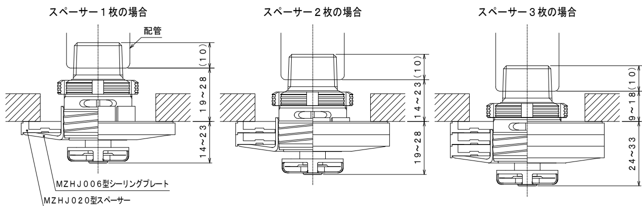
図 8. スペーサー使用時の取り付け状態（シーリングプレート）
