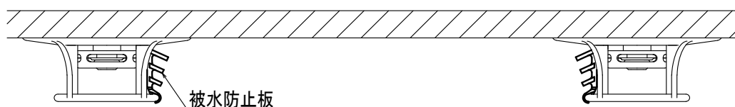
図 13. 被水防止板の取り付け（その 2）
