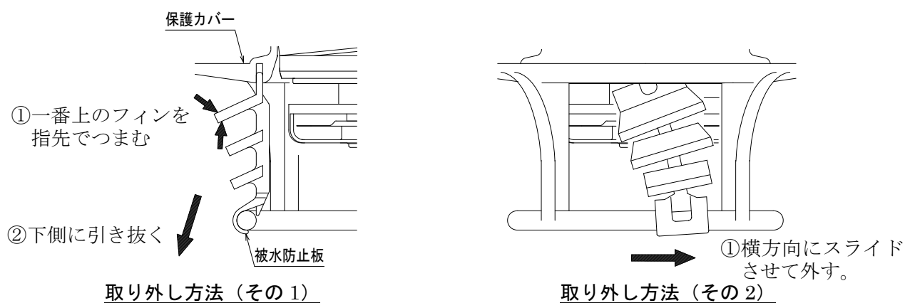
図 14. 被水防止板の取り外し
