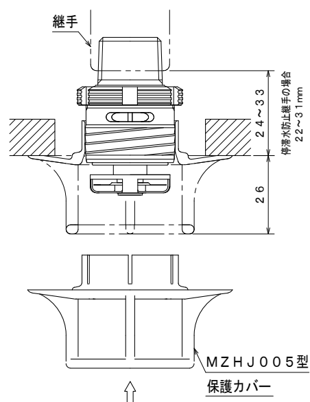
図 10. 保護カバーの取り付け
