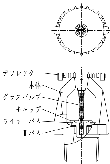
図 1. 外観図
