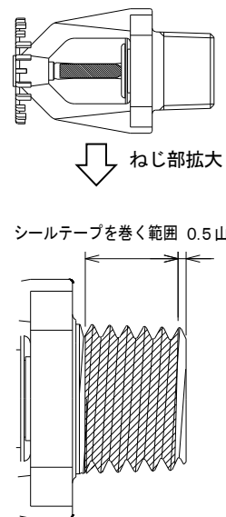
図 5. シールテープの巻き方
