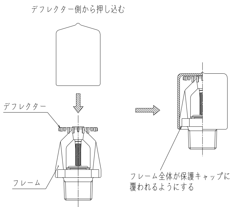
図 6. 保護キャップの取り付け
