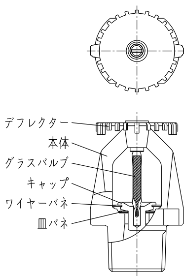
図 1. 外観図
