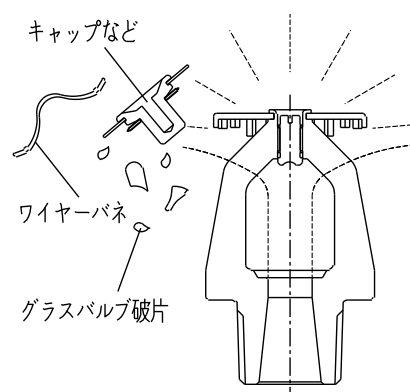
図 2. 作動状態図
