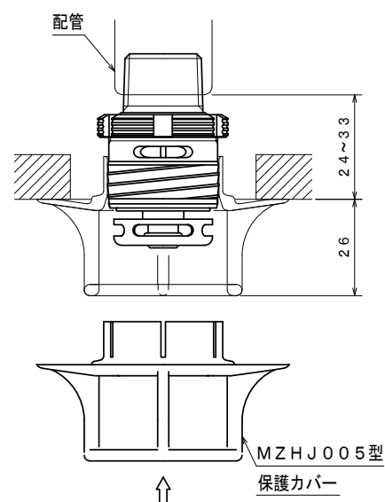
図 8. 保護カバーの取り付け
