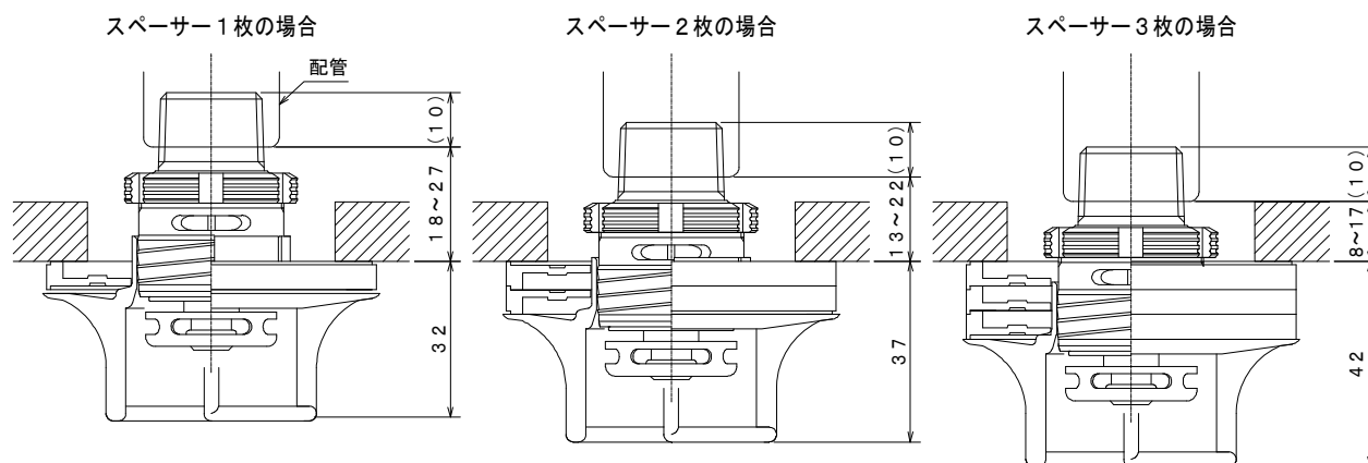
図 9. スペーサー使用時の取り付け状態（保護カバー）
