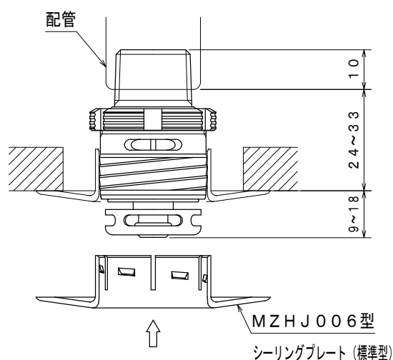
図 5. シーリングプレートの取り付け
