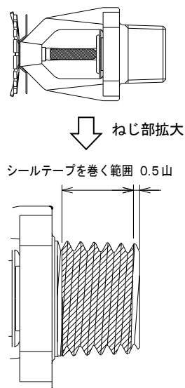
図 5. シールテープの巻き方
