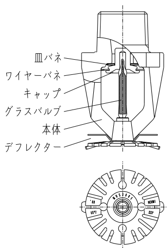
図 1. 外観図
