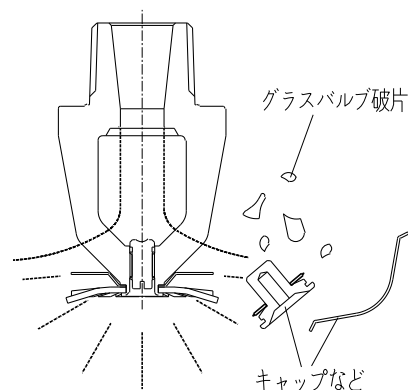
図 2. 作動状態図
