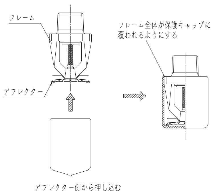
図 6. 保護キャップの取り付け
