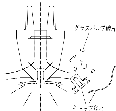
図 2. 作動状態図
