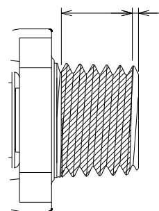
図 5. シールテープの巻き方
