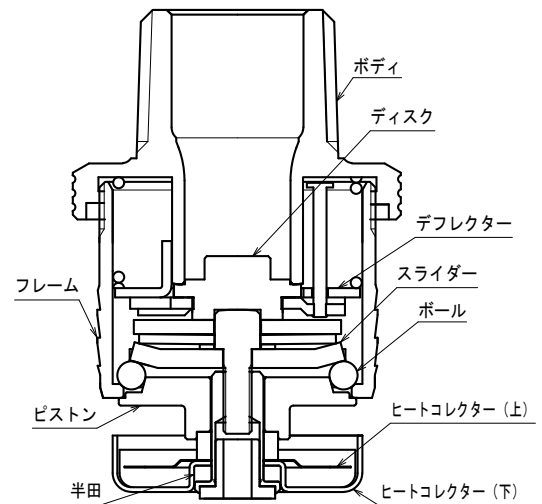
図 1. 構造図
