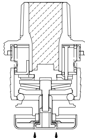
図 2. 作動状態図
