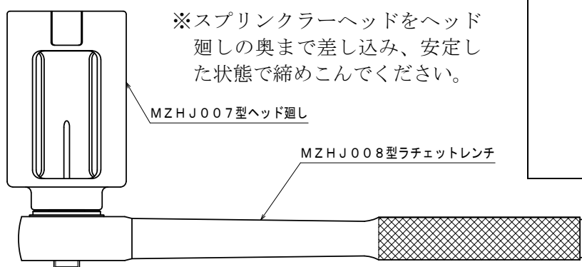
図 3. スプリンクラーヘッド取付図
