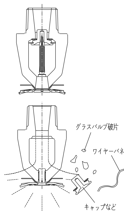
図 2. 作動状態図
