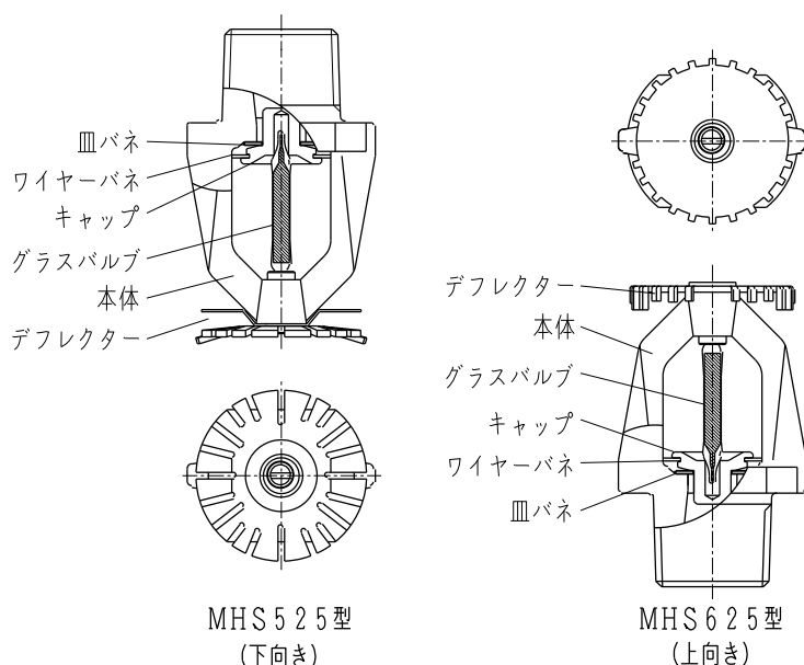
図 1. 外観図
