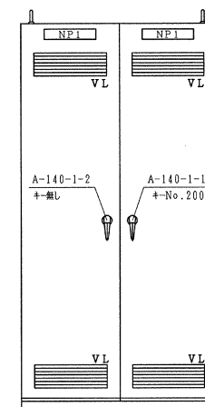
背面図 (1/20)
