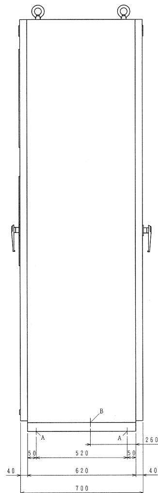
右側面図
