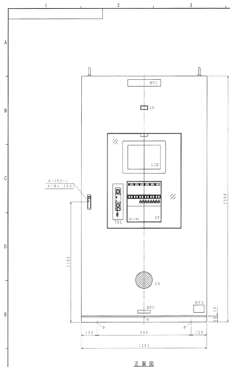
正面图
