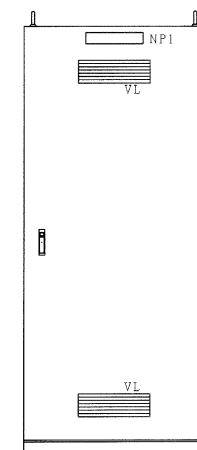
背面図 (1/20)
