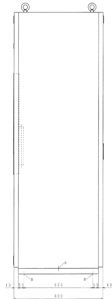
側面図
