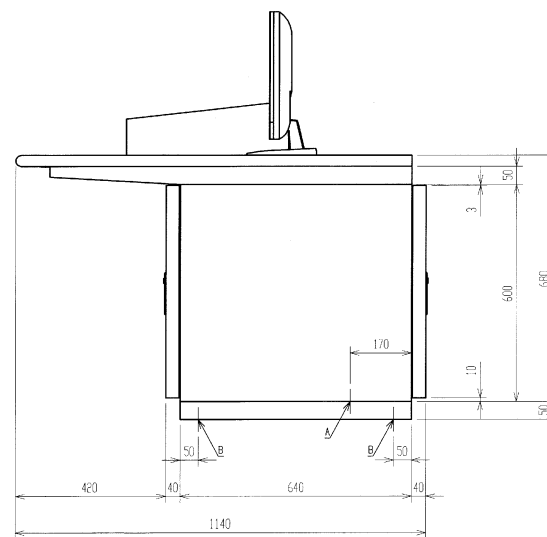
右側面図
