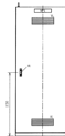
背面図 (1 / 20)
