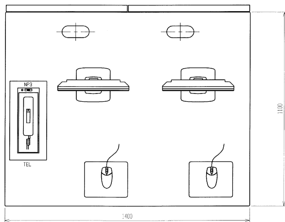
平面図
