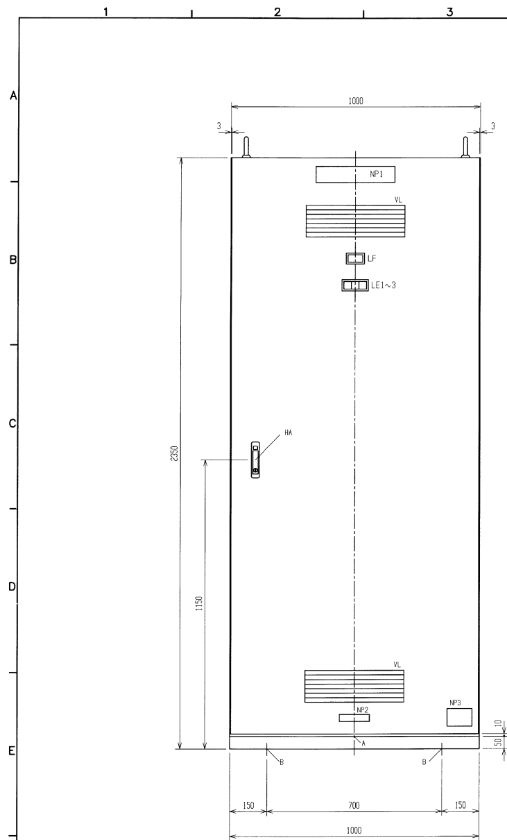
正面图
