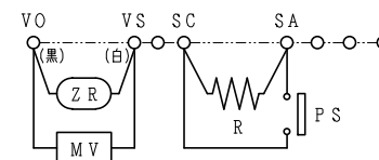
結線図
