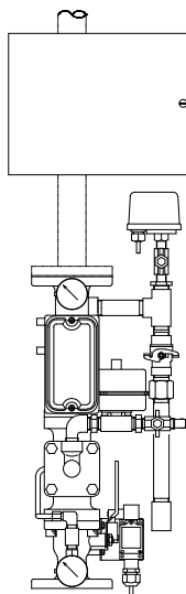
MAJ043B 型
